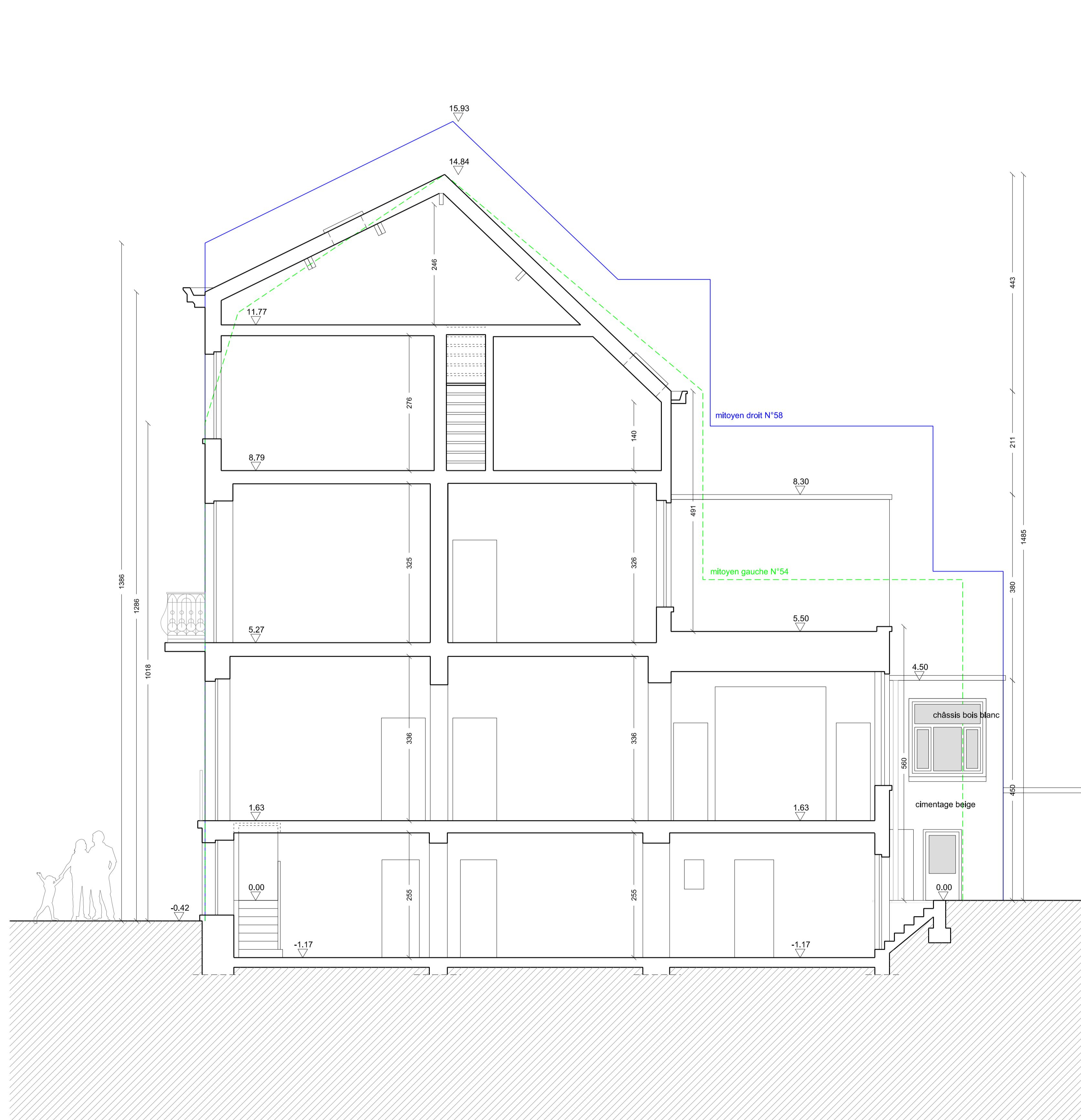
Coupe A
